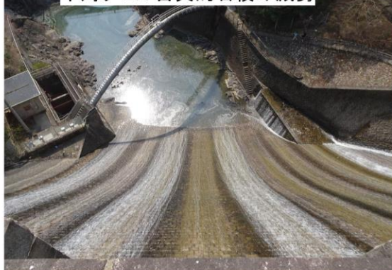
千苅ダム：古典的石積み減勢
