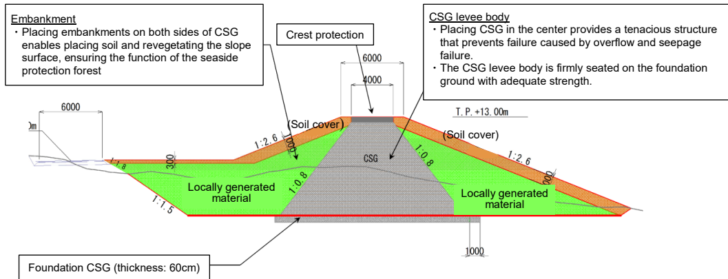
Fig. 2 Typical cross section of the coastal levee Coupe trancheversale typique de la digue côtière
