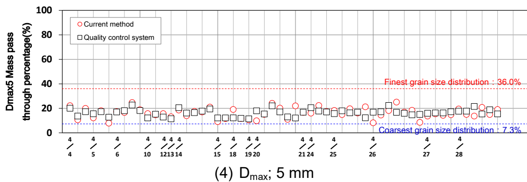
Fig.21 Temporal change of grain size distribution (Comparison of two measuring method using same material) Variation temporelle de la distribution de taille de grain (Comparaison de deux méthodes utilisant le même matériel de mesure)
