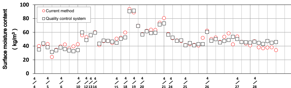
Fig. 20 Temporal change of surface moisture content Variation temporelle de teneur en humidité de surface
