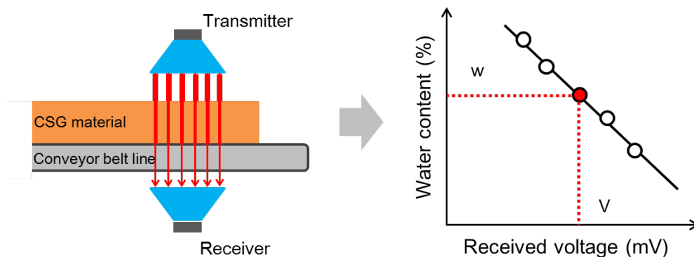
Fig. 18 Microwave moisture meters and their measuring principal Appareils de mesure de l'humidité à micro-ondes et leurs principales mesures
