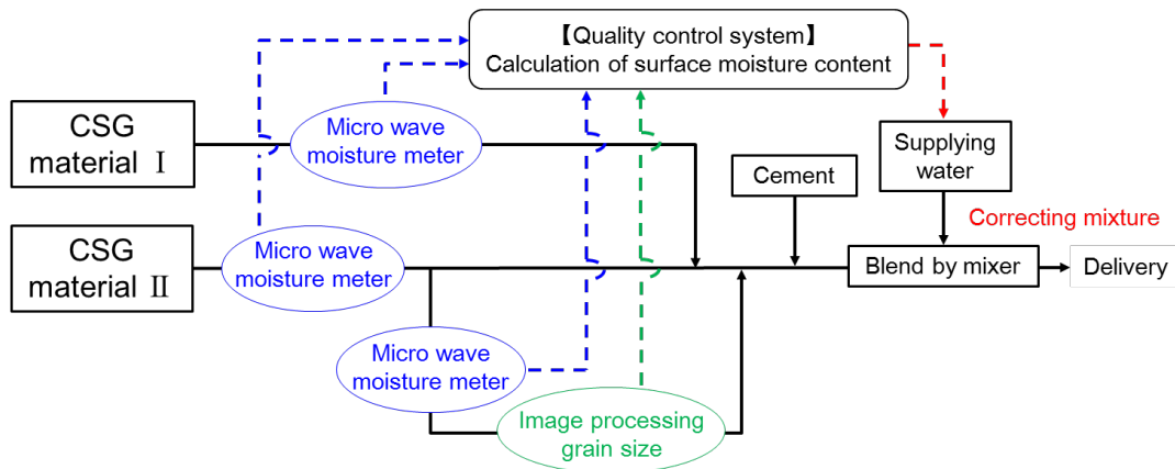
Fig. 15 Quality control system Système de contrôle qualité
