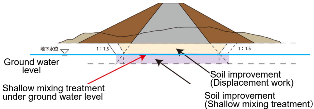
Fig. 13 Soil stabilization method and depth of stabilization Méthode de stabilisation de sol et profondeur de la stabilisation
