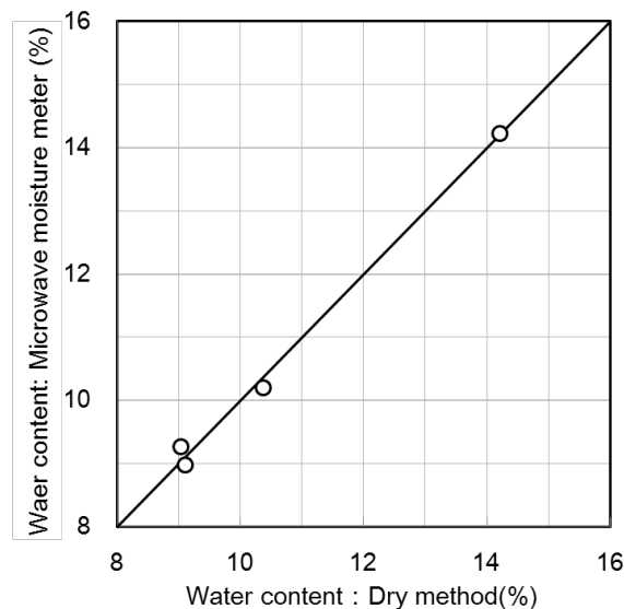
Fig .19 Calculation of water content by two different methods Calcul de la teneur en eau par deux méthodes différentes
