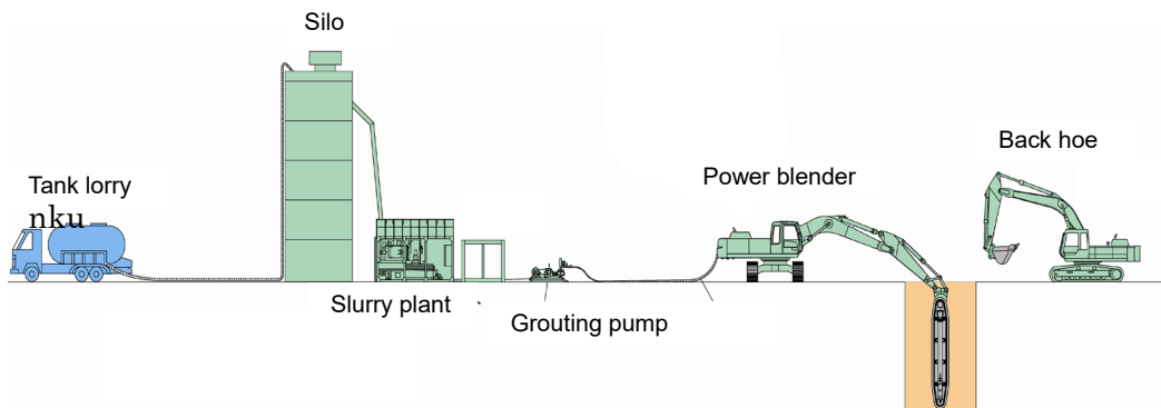
Fig. 14 Equipment of soil stabilization and its arrangement Équipement de la stabilisation des sols et arrangement
